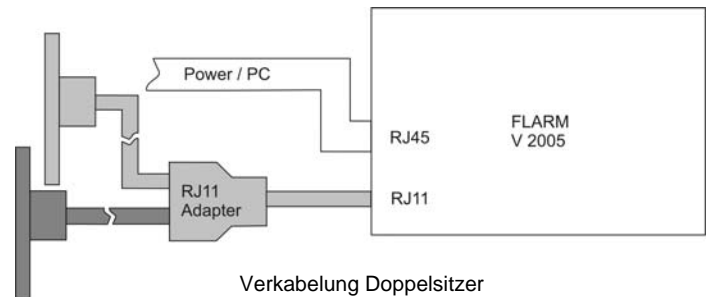
Verkabelung Doppelsitzer
