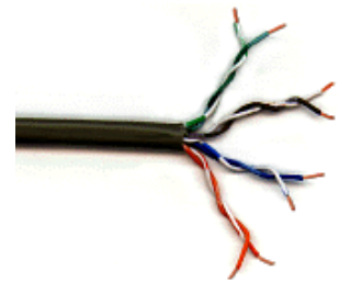
Offenes Ende Patchkabel
